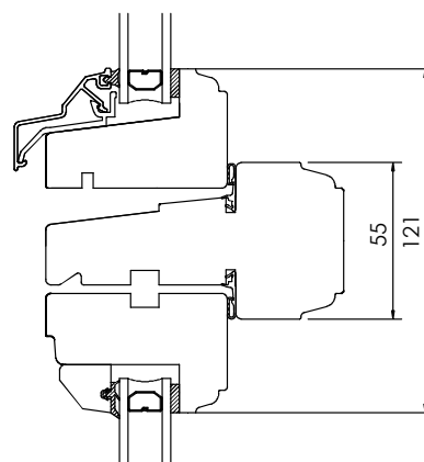
Vertikalsnitt 2-luft Vertical section 2-lights
