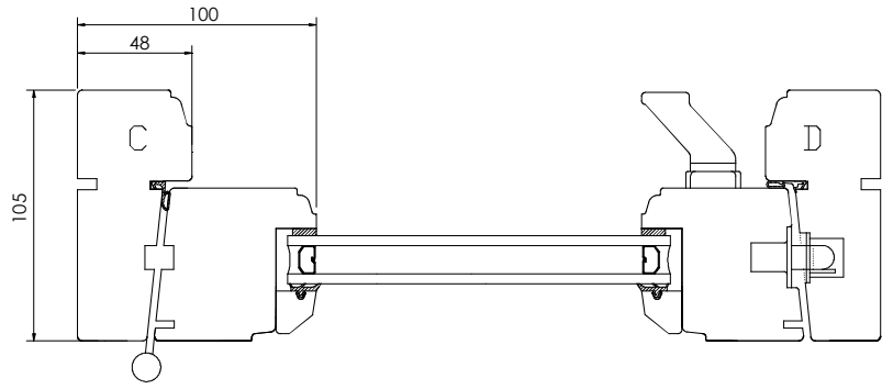
Horizontalsnitt Horizontal section
