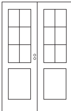
PARDÖRR 13,3 625+625 mm
