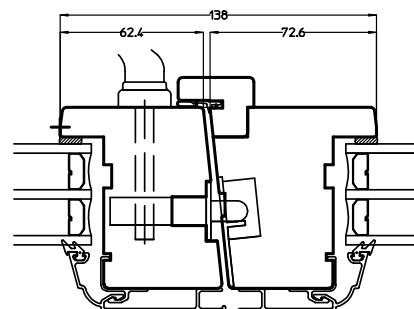
Horizontalsnitt mötesbåge
