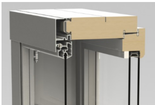
Fönstersnitt
